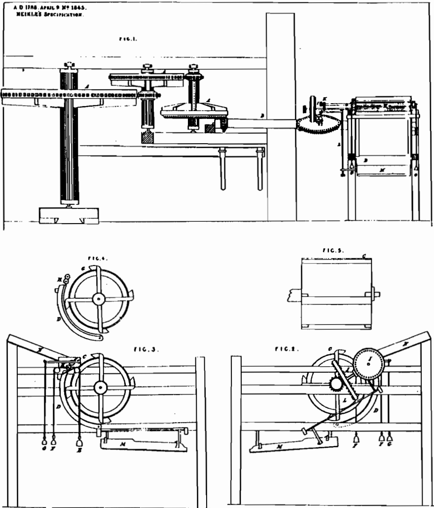
Fig. 1. — La machine à battre les grains d'Andrew et George Meikle. D'après le brevet Meikle de 1788. Les organes accessoires, secoueur, grille, etc., destinés à séparer le grain de la paille après le battage proprement dit, ne sont pas représentés.
