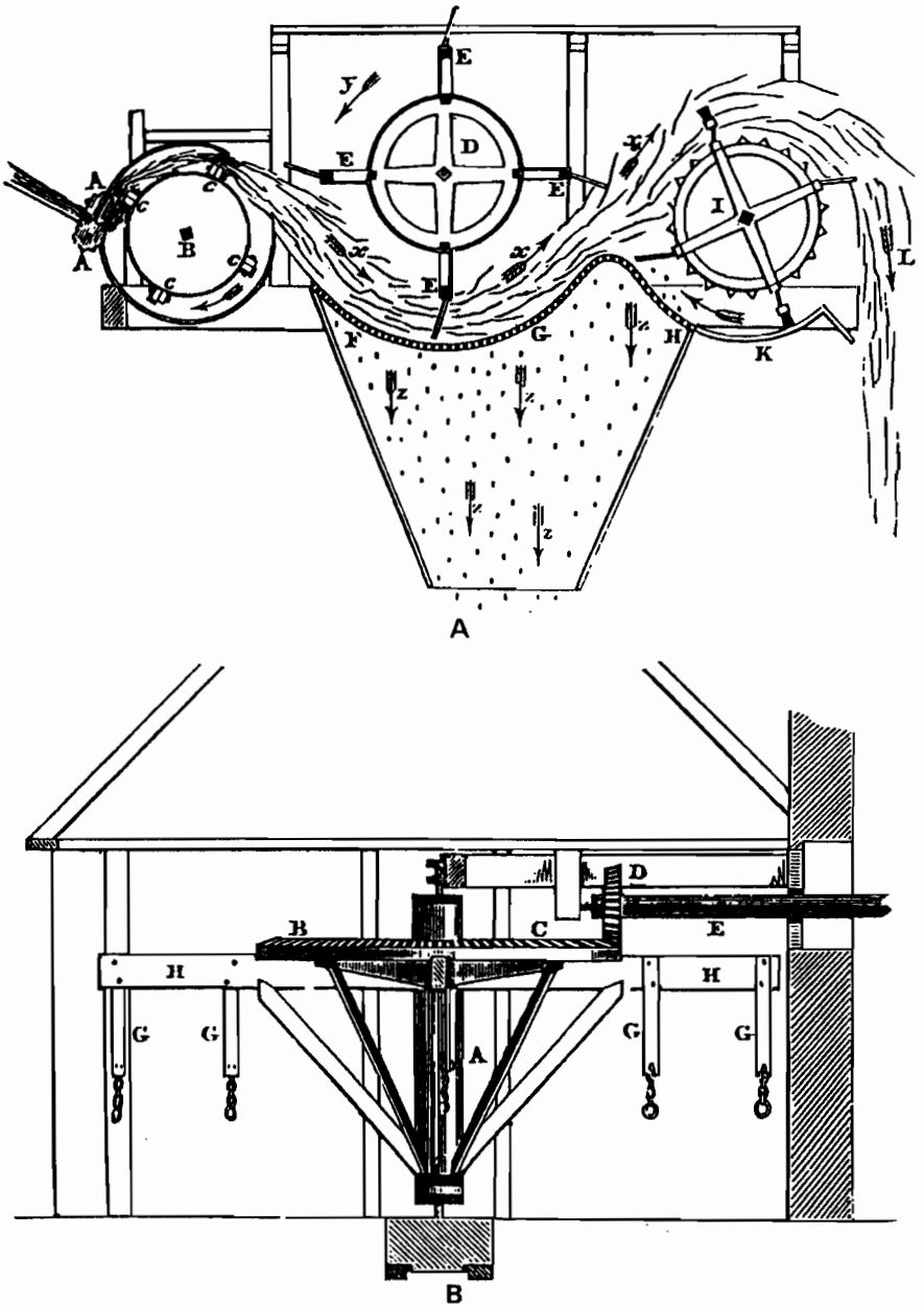
Fig. 2. — La machine à battre les grains d'Andrew et George Meikle. D'après une gravure de 1840. La machine est complète, avec ses organes accessoires. Source : A. Fenton, Scottish Country Life , Édimbourg, John Donald, 1976.
