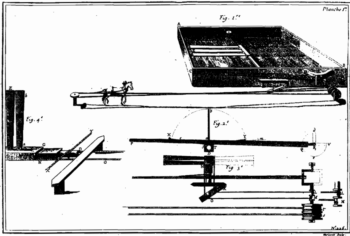
Fig. 3. — La machine à battre de Du Quet (1722).
